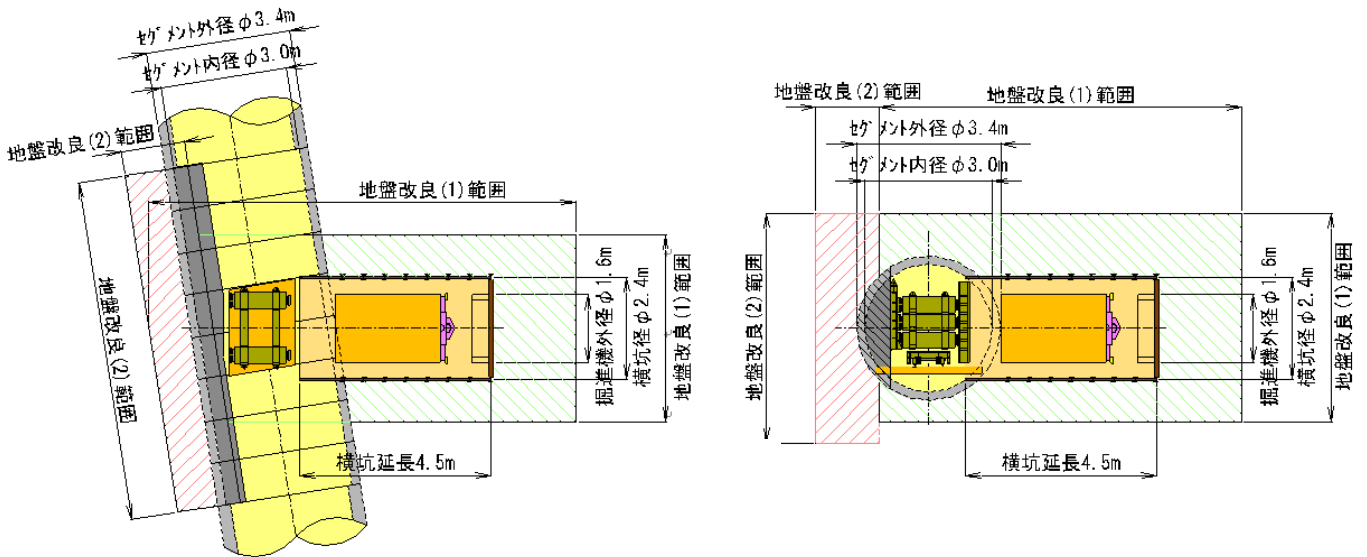
図-6 発進部の仮設計画
